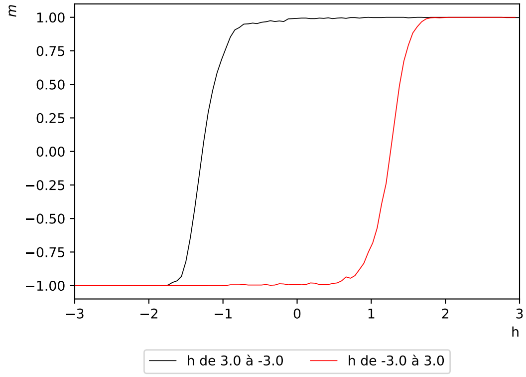
Hystérésis de l'aimantation - réseau de taille L=32 - champ magnétique d'amplitude h=3 à T=1.5
